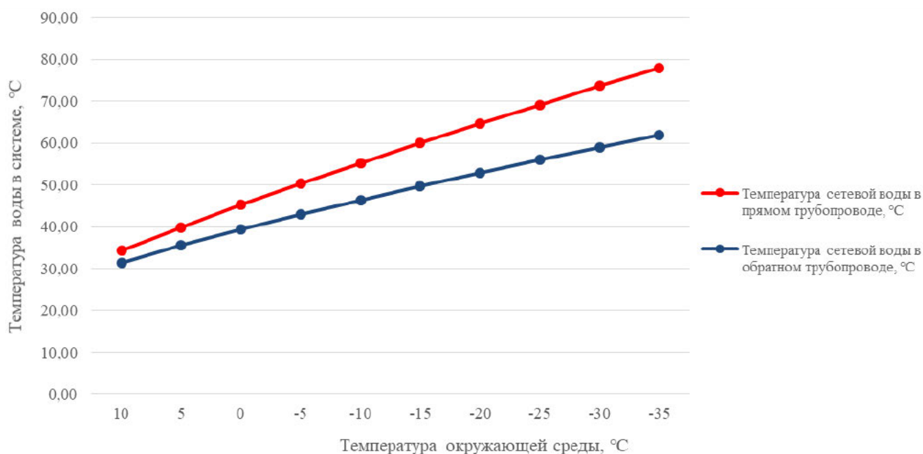
Рисунок 2.2 – График изменения температур теплоносителя котельной (температурный график 78/62°С)
